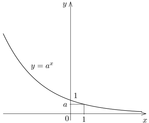
0 < a < 1 のときの y = a^x のグラフ
